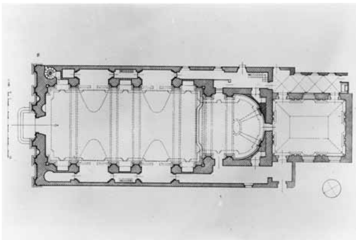
87. Cuneo, S. Maria, Grundriss.
