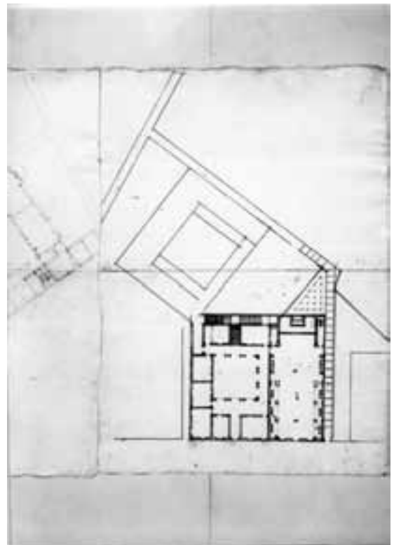
95. Genua, Kolleg, Plan Nr. 7, Entwurf für Kirche und Schultrakt.
