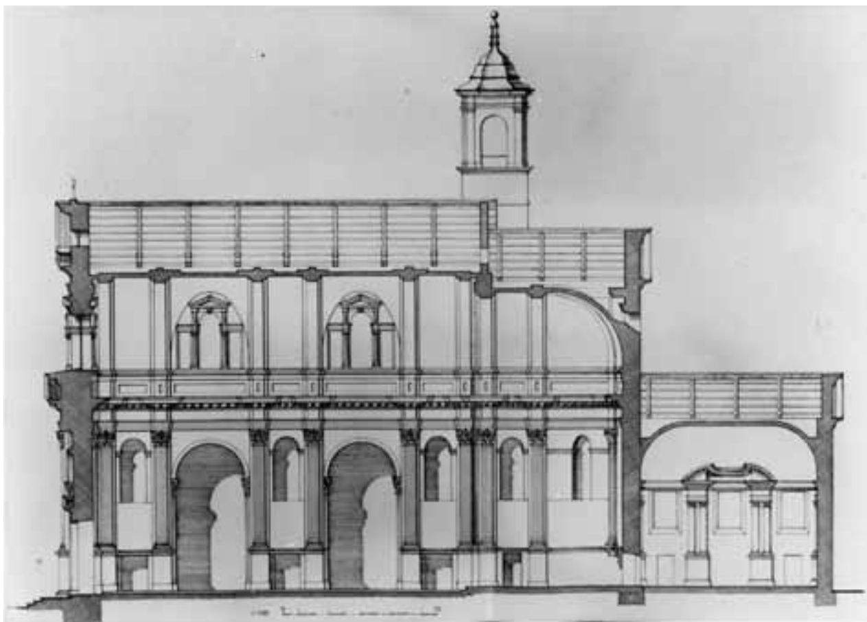
85. Cuneo, S. Maria, Längsschnitt.
